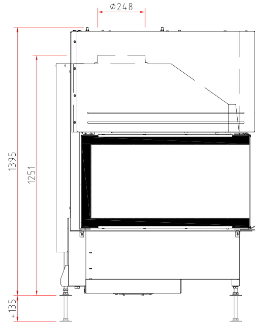
Seitenansicht M 1:20
